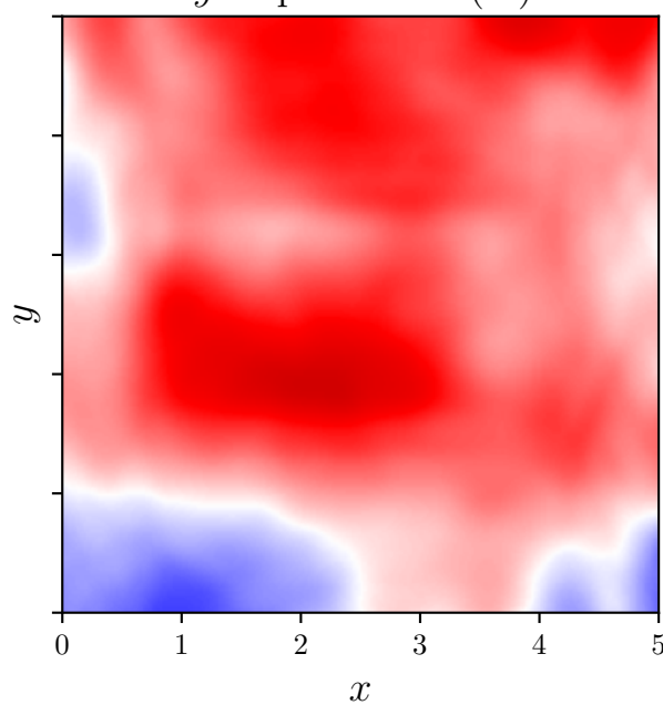
Final y displacement (m) id=0
